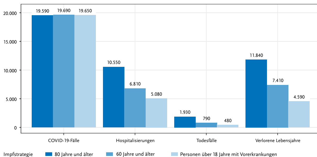
Abb. 12 | Kumulativer Impact von COVID-19-Impfstrategien bis 12 Wochen nach Impfstart (Basis-Szenario)
