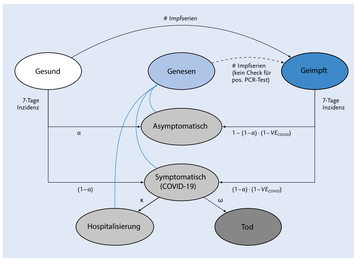
Abb. 10 | Schematische Darstellung des Markov Modells zur Berechnung der direkten Impfeffekte auf Bevölkerungsebene
