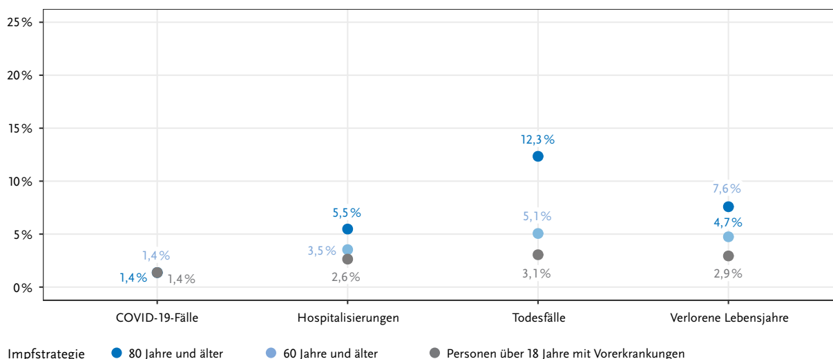
Abb. 13 | Relativer Impact von COVID-19-Impfstrategien bis 12 Wochen nach Impfstart (Basis-Szenario)
