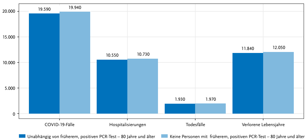
Abb. 14 | Impact von COVID-19 Impfstrategien (Szenario Ausschluss von Personen mit SARS-CoV-2-PCR-Nachweis in der Anamnese)
