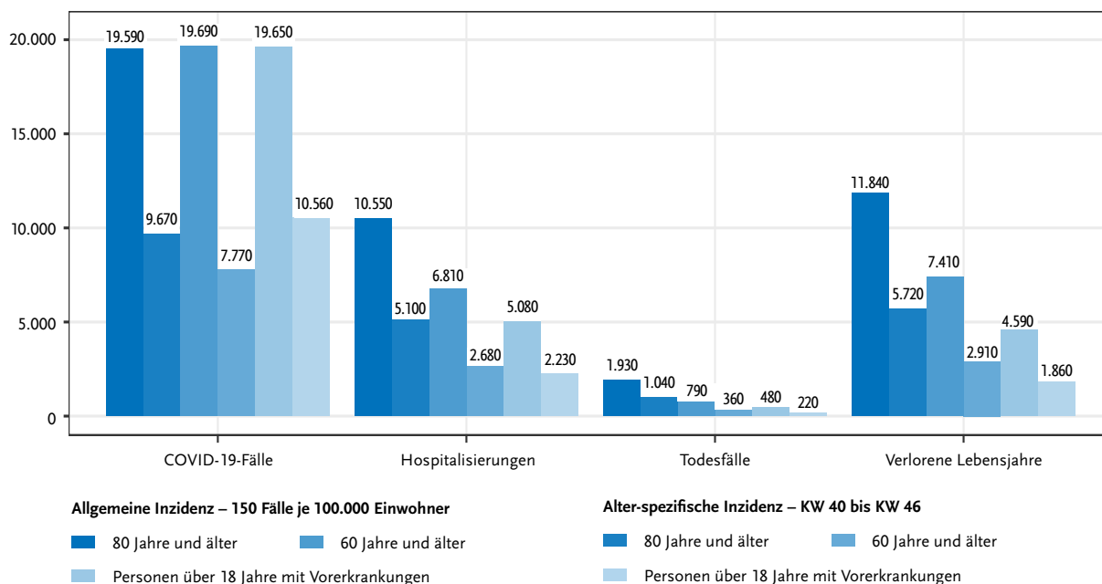
Abb. 15 | Kumulativer Impact von COVID-19-Impfstrategien bis 12 Wochen nach Impfstart (Szenario Infektionsgeschehen)
